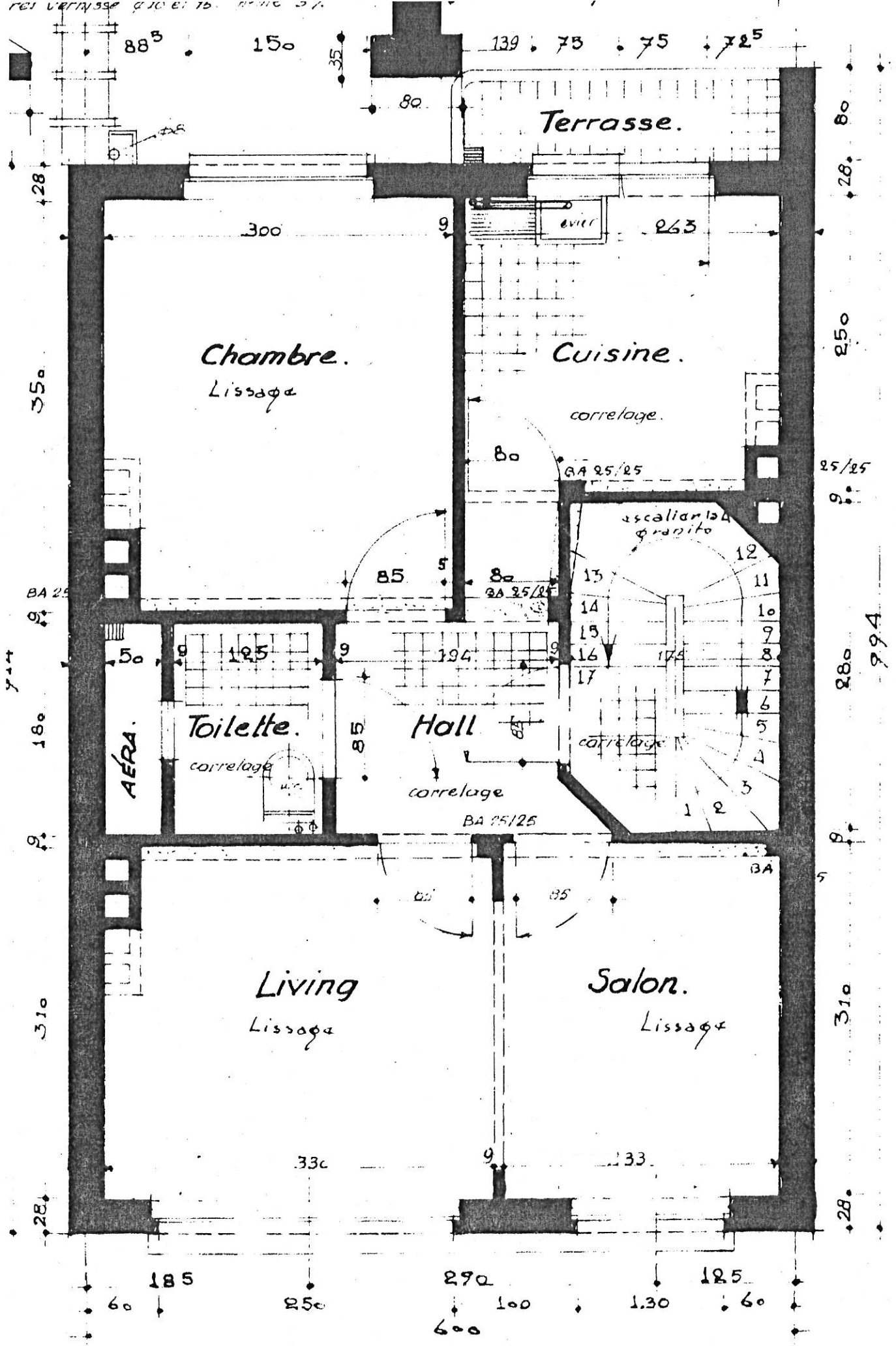
Etage Normal. 1.2.3.
